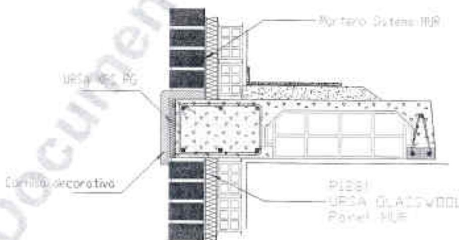
Figura 3: Frente de forjado. Corrección de puente térmico en frente de forjado
