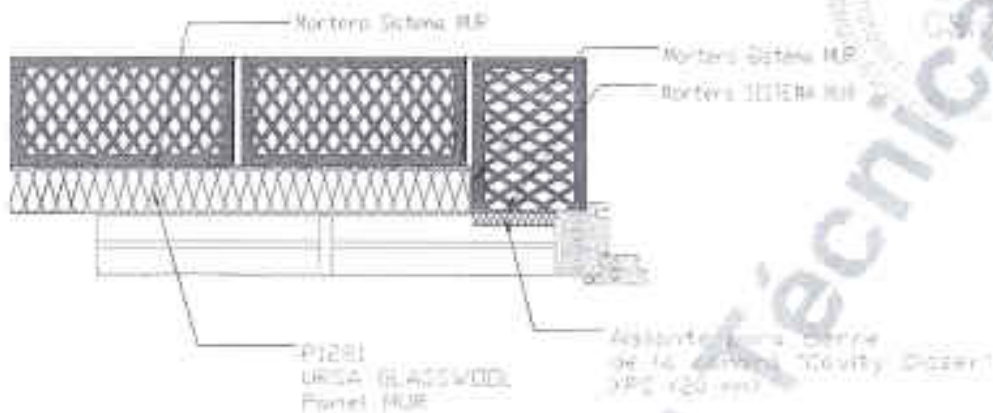
Figura 5: Jambas en ventana con corrección de puente térmico mediante carpintería
