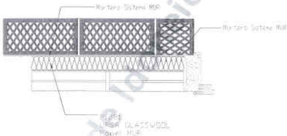
Figura 6: Antepecho de ventana
