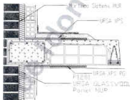
Figura 3: Frente de forjado. Corrección de puente térmico en frente de forjado
